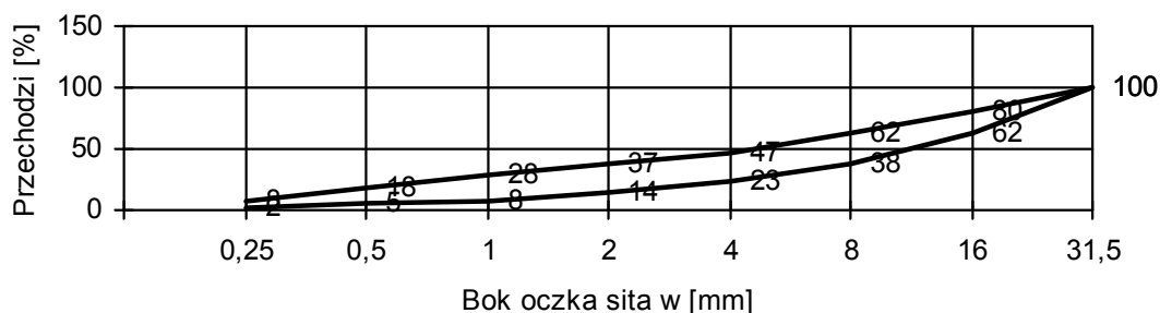
Krzywa uziarnienia kruszyw 0 - 31.5 mm
